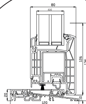
Aluminium onderdorpel
