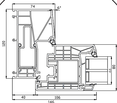
Zijstijl
