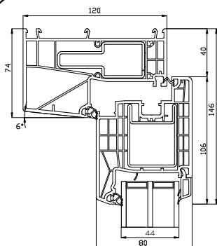
Bovendorpel
