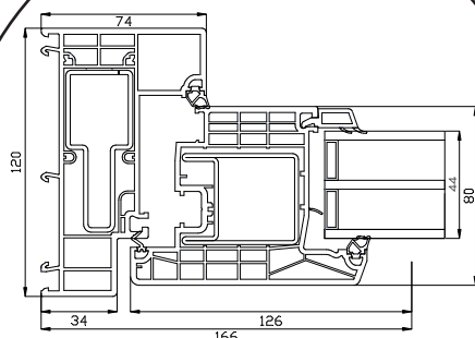
Zijstijl
