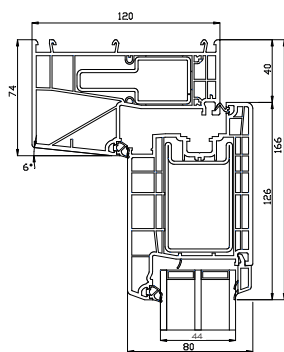
Bovendorpel
