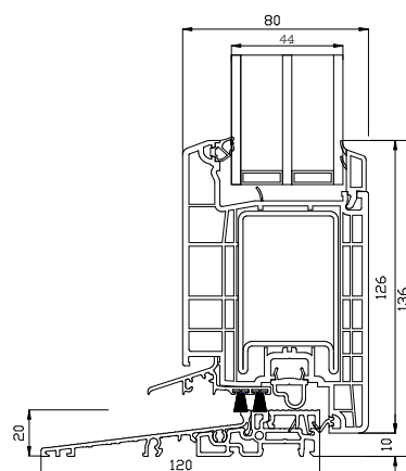
Onderdorpel
