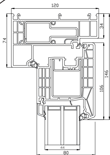
Bovendorpel
