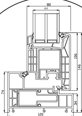
Kunststof onderdorpel
