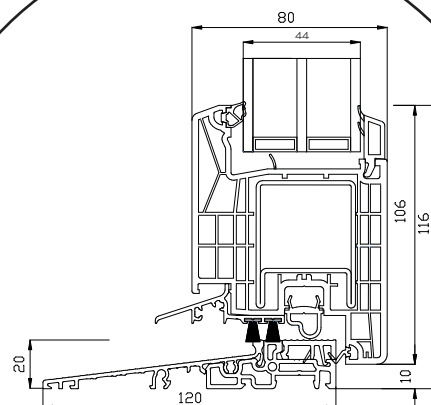
Aluminium onderdorpel
