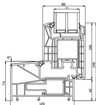
Kunststof onderdorpel
