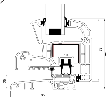
Dørterskel i aluminium
