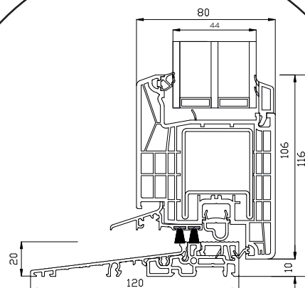
Aluminium onderdorpel
